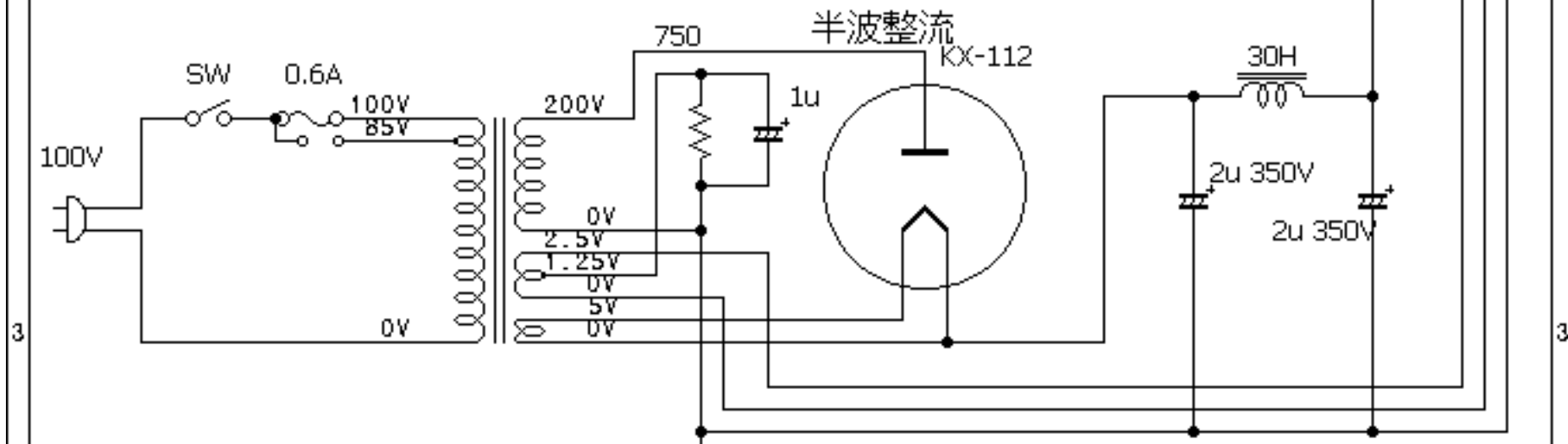
カセドラル並三受信機回路図 2007.12.10 Y.KONDO
